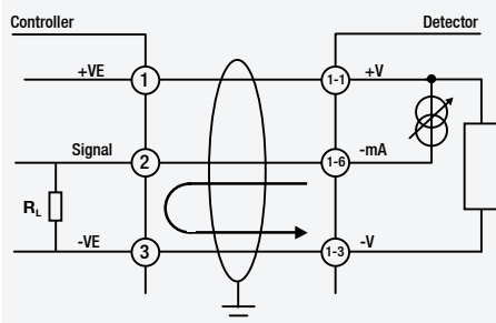
Configuration en émetteur du XXN
