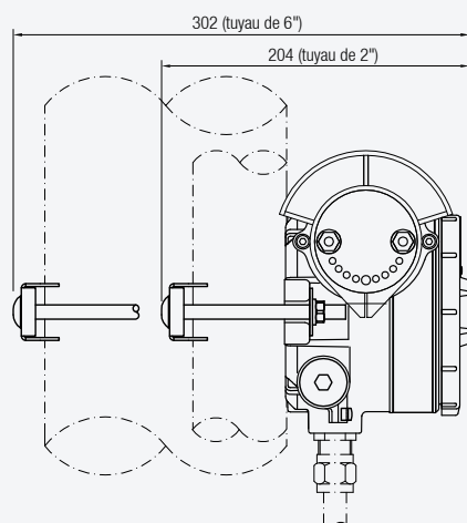
Montage sur tuyau
