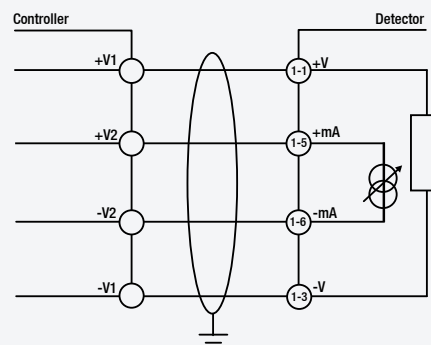
Configuration en isolé du XXN
