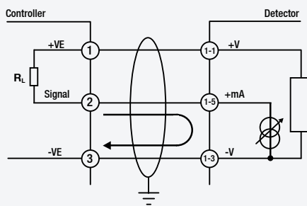
Configuration en récepteur du XXN
