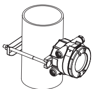
Vertikale oder horizontale Rohrmontage (unter Verwendung der optionalen Rohrmontagehalterung)
