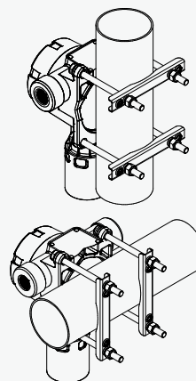
Vertikale oder horizontale Rohrmontage (unter Verwendung der optionalen Rohrmontagehalterung)
